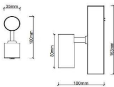
UMAG-SPOT5
