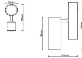
UMAG-SPOT12
