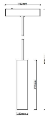
UMAG-PENDANT10
