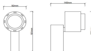
UMAG-SPOT15
