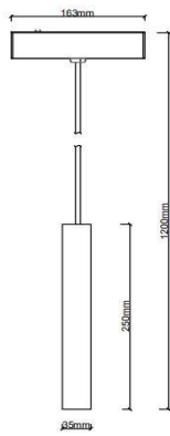
UMAG-PENDANT5
