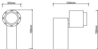
UMAG-SPOT8
